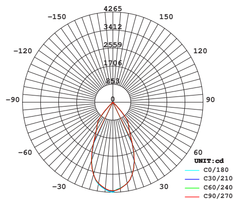
Lichtstärkeverteilung FraS
