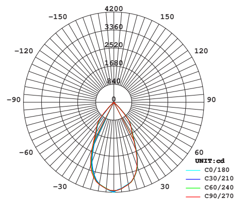
Lichtstärkeverteilung FraR
