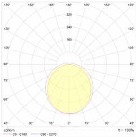
Polardiagramm 120°
