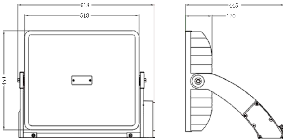
Abmessungen PLUTO (mm)
