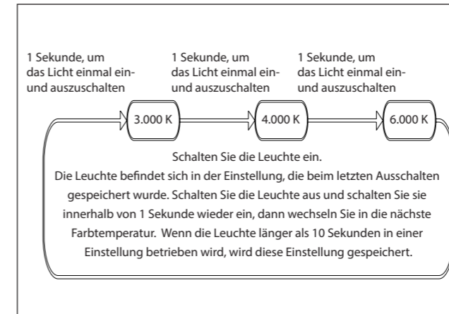
Abb. 7: Wahl der Farbtemperatur über Aus- und Einschalten der Leuchte.
