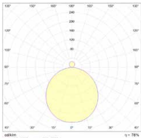
Polardiagramm
