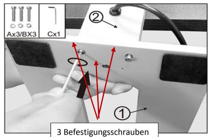
Abb. 3: Anschrauben des Standfußes
