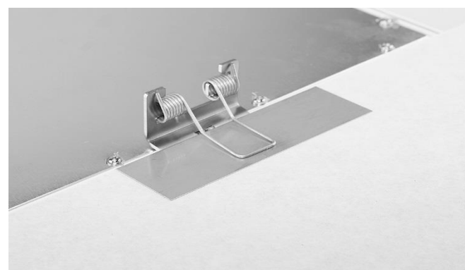
Abb. 8: Ansicht des Federbügels in der Decke
