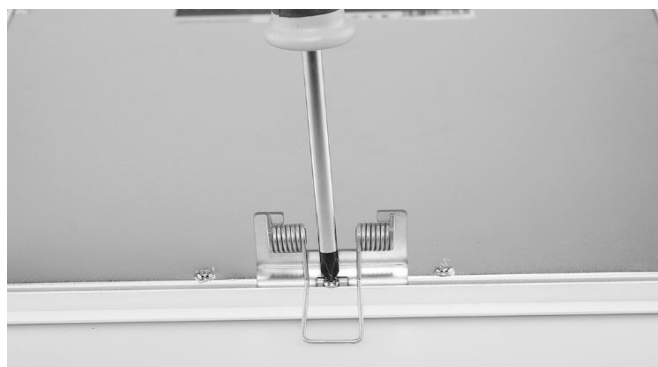
Abb. 7: SNAP-IN Federbügel für LED Panel SNAP Frame-In-One
